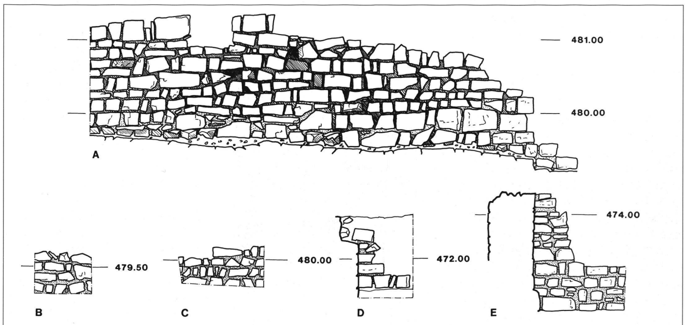
4: Mauerstrukturen, Massstab 1:50.
