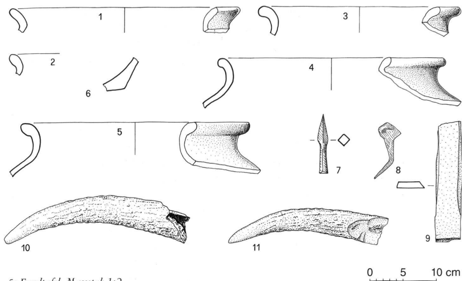
5: Fundtafel, Massstab 1:2.
