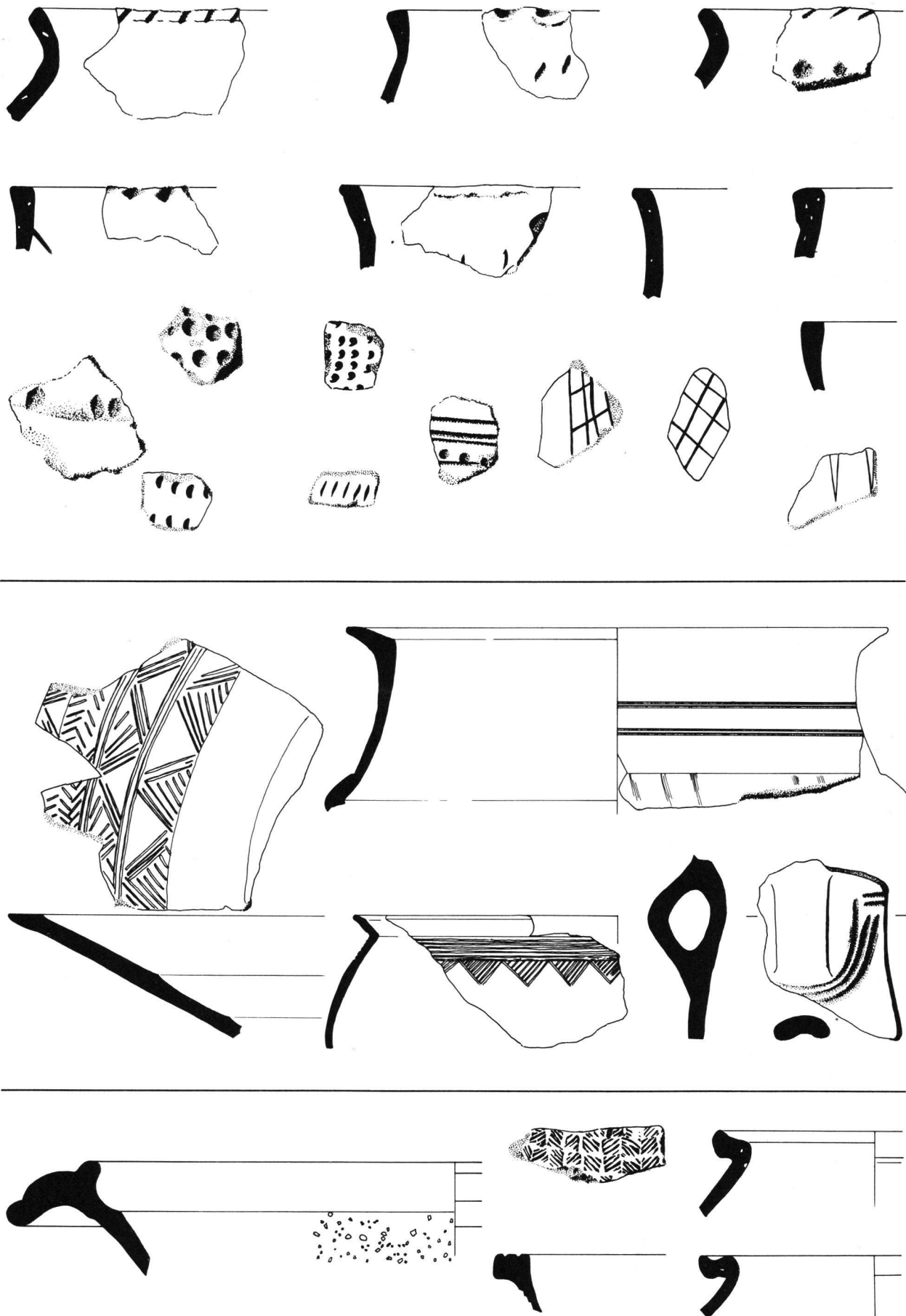
Trimbach-Frohburg, Keramik. Oben: Mittlere Bronzezeit. Mitte: Späte Bronzezeit. Unten: Römerzeit, Massstab 1 : 2
