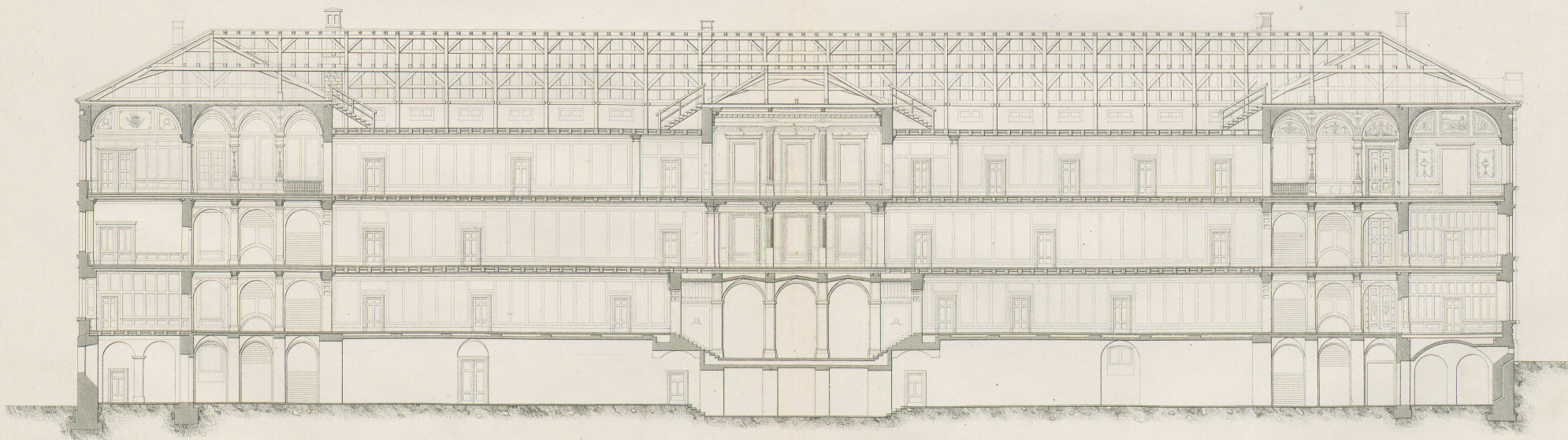
Längenschnitt durch die Mitte des Gebäudes
