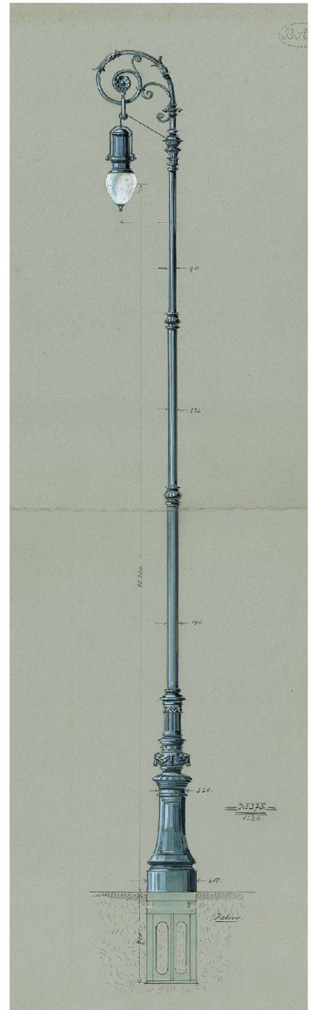
Abb. 8 a: Candelaber mit Bischofsstab für electriche Bogenlampe; b: Candelaber für Bogenlampe; c: ohne Beschriftung, um 1910 (Klosterarchiv Einsiedeln, Plan 3.138.0002).
