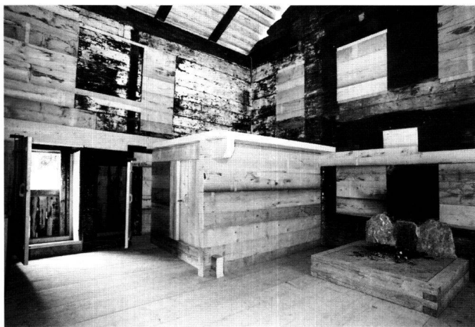
Abb. 6: Schwyz: Haus am Landsgemeindeplatz, Hinteribach – heute im Freilichtmuseum Ballenberg. Die Küche mit der offenen Feuerstelle und der rekonstruierten Kammer in der Nordwestecke. Links davon die originalen Türöffnungen zur Laube und zur Abortanlage.
