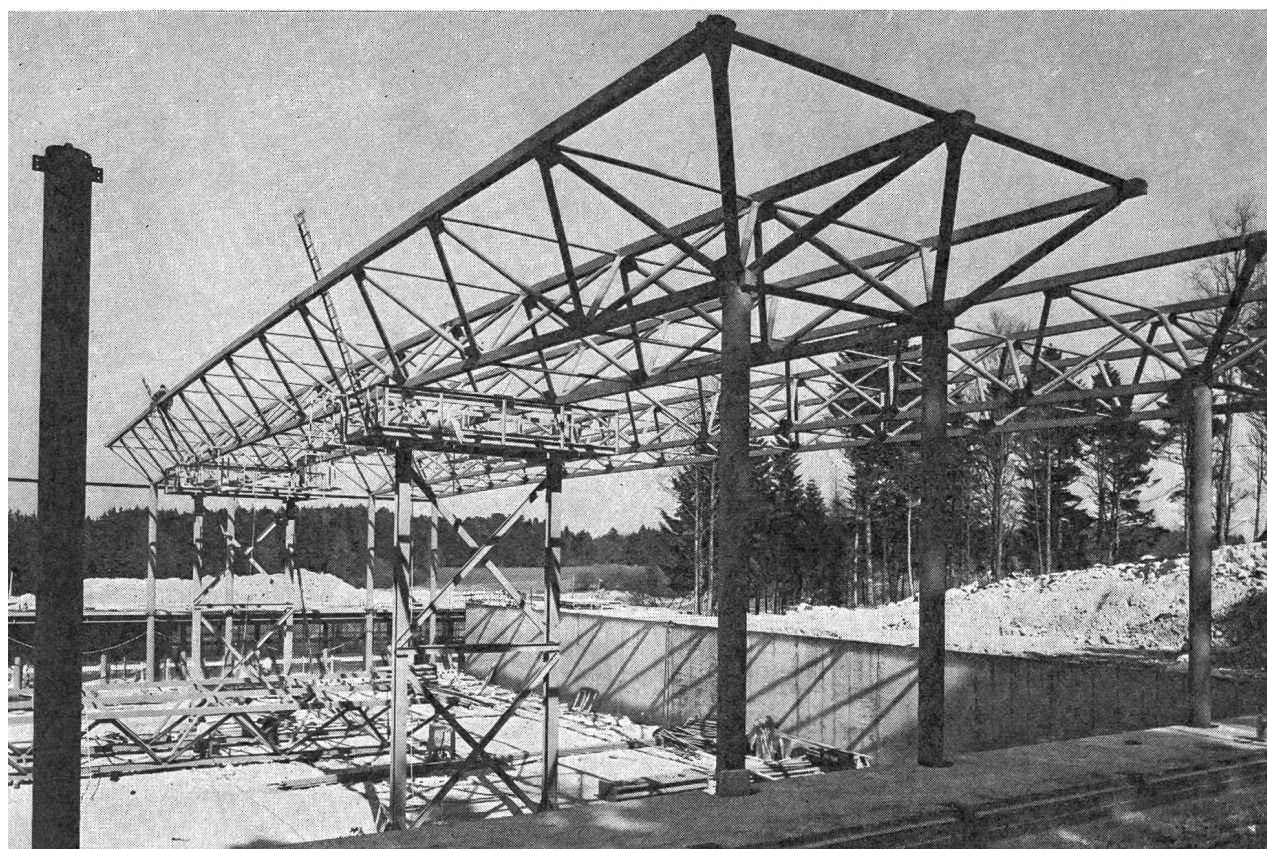
Montage des immenses porteurs métalliques en juin 1975 – une opération délicate et spectaculaire. La moindre faute peut avoir des conséquences catastrophiques.
