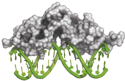
Proteine wirken auf die DNA ein
