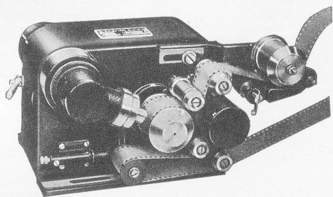
Klangfilm „Europa“-Lichttongerät
