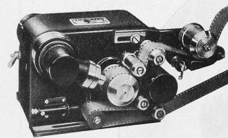
«Europa»-Lichtongerät Lecteur de son «Europa»
