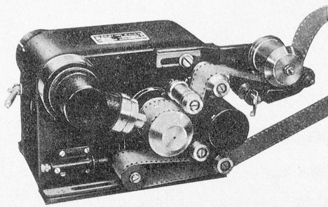
„Europa“ Lichttongerät
