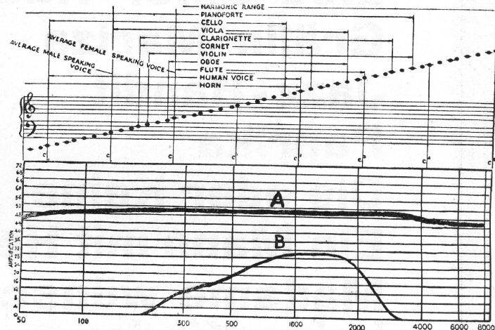
A Courbe de notre installation B Courbe d'une installation ordinaire
