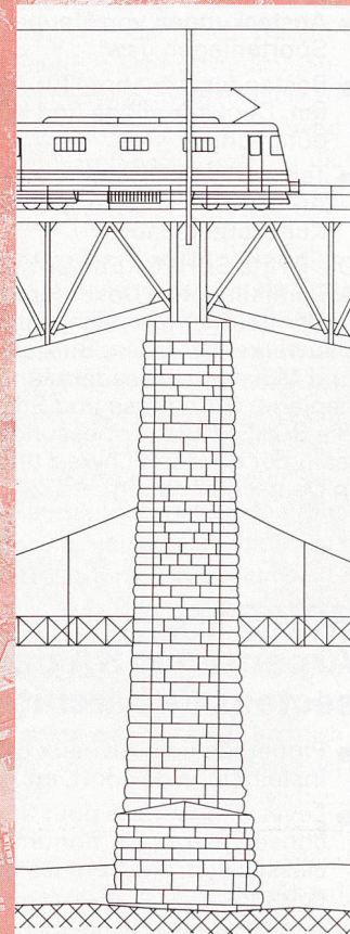
Photogrammetrische Auswertung Evaluation photogrammétrique
