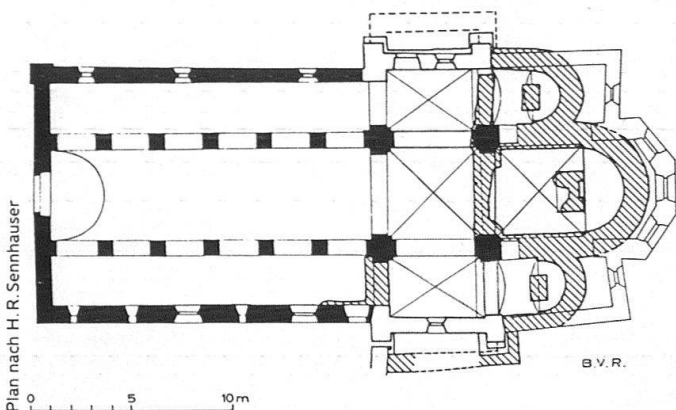
Rougemont, Kirchengrundriss
