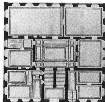
Fig. 3. Neuchâtel. Ancien Hôtel Bellevue en 1978. – Plans d'après 28 e réunion des architectes, 1879. Rez-de-chaussée (en bas) et 1 re étage
