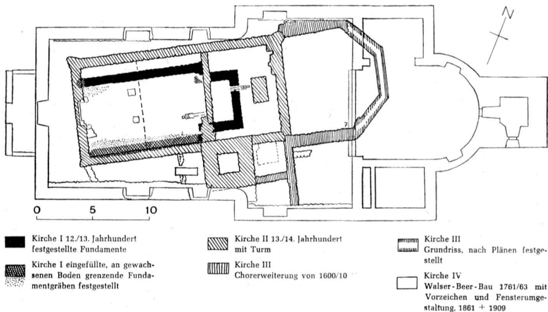
Ausgrabungsgrundriß der Kirche von Niederbüren
