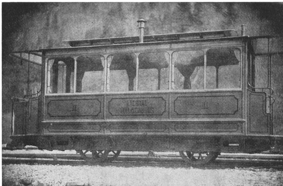
WB-Personenwagen 2. Klasse mit 18 Sitzplätzen, Eigengewicht 2300 kg.
