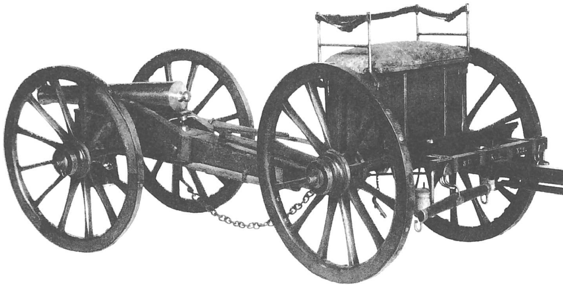
Abb. 4: Sechspfünder-Kanone Modell 1843, aufgeprotzt mit Protze (rechts) und Deichsel. Die Wirkung der Artillerie war begrenzt. Man schoss auf Sicht über das Rohr. Bei einer mittleren Distanz von 300 Metern trafen nur 15 Prozent der Schüsse. Aus Betschmann, Walter: Geschütze der Artillerie ohne mechanischen Rohrrücklauf. Bewaffnung und Ausrüstung der Schweizer Armee seit 1817, Band 8, Dietikon-Zürich 1980, S. 62.
