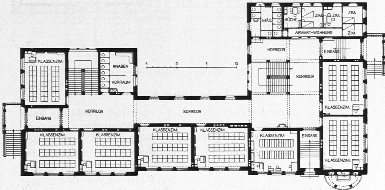
Heiligbergerschulhaus: Erdgeschoß.
