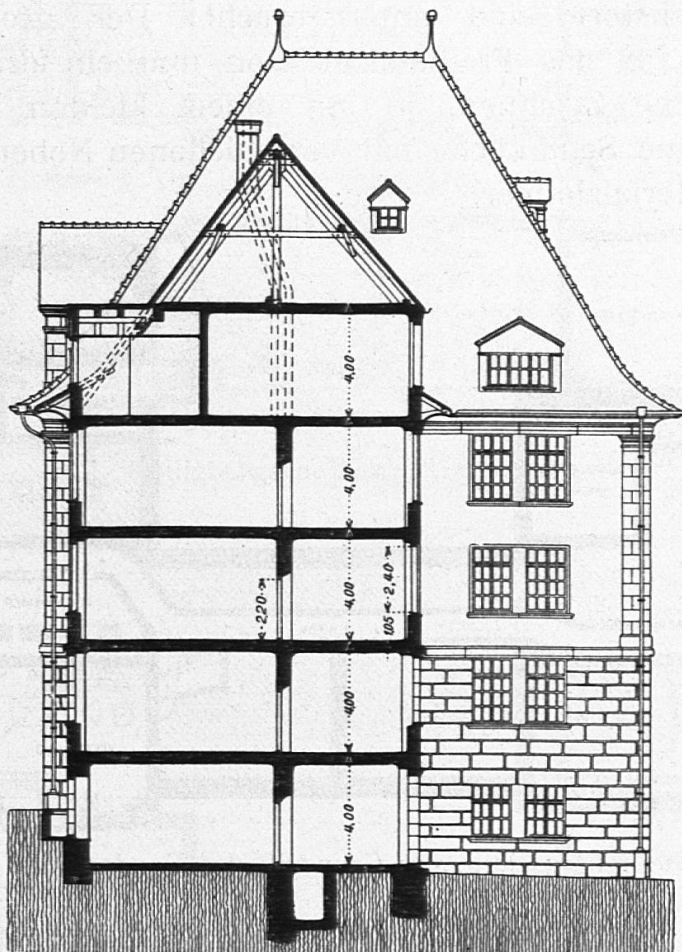
Heiligbergschulhaus: Querschnitt.
