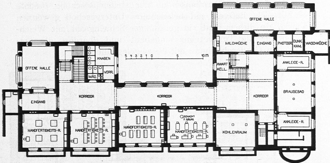
Heiligbergerschulhaus: Untergrundgeschoß.
