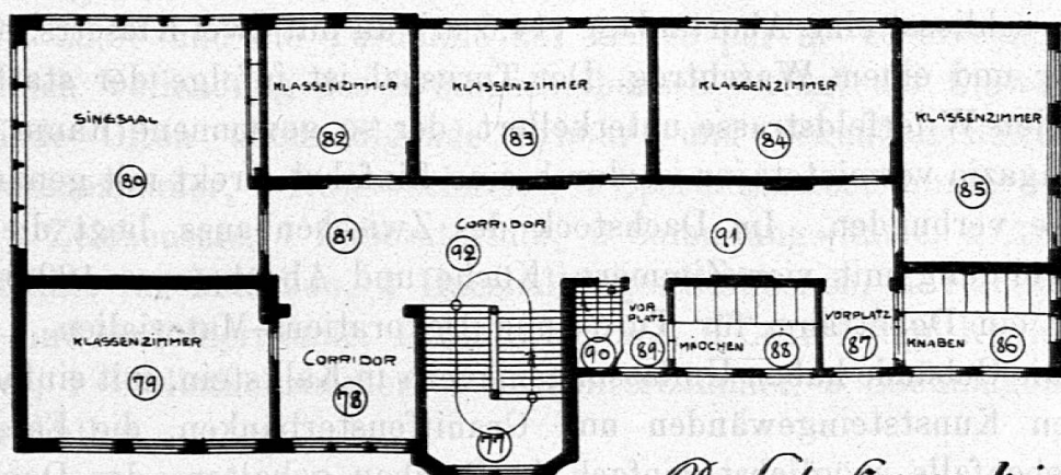
Dachstockgrundriss.
