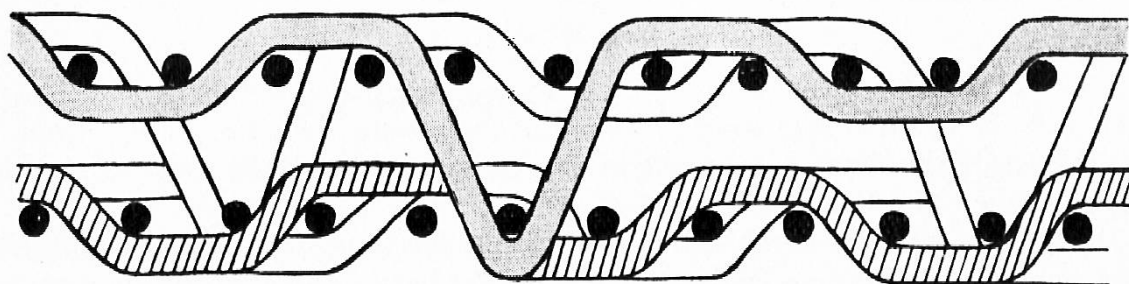
DOPPELGEWEBE
