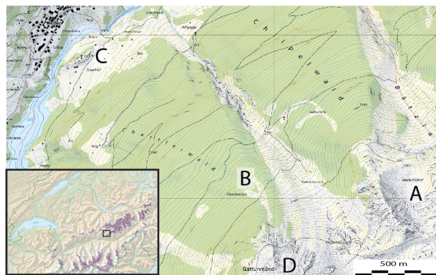
Fig. 2. Lötschental, VS. Le versant nord du Bietschorn au sud du village de Kippel. A : « Bätzlerfriedhof ». B : « Chastlerbord ». C: colline « Chastel ». D: « Gattunmandli ». Carte Swisstopo.
