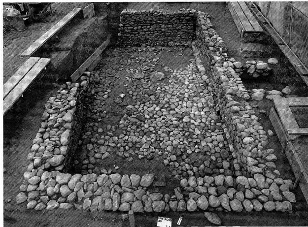
Fig. 20. Cressier FR, Route des Roches. Cave avec entrée latérale condamnée lors de l'agrandissement du local.
