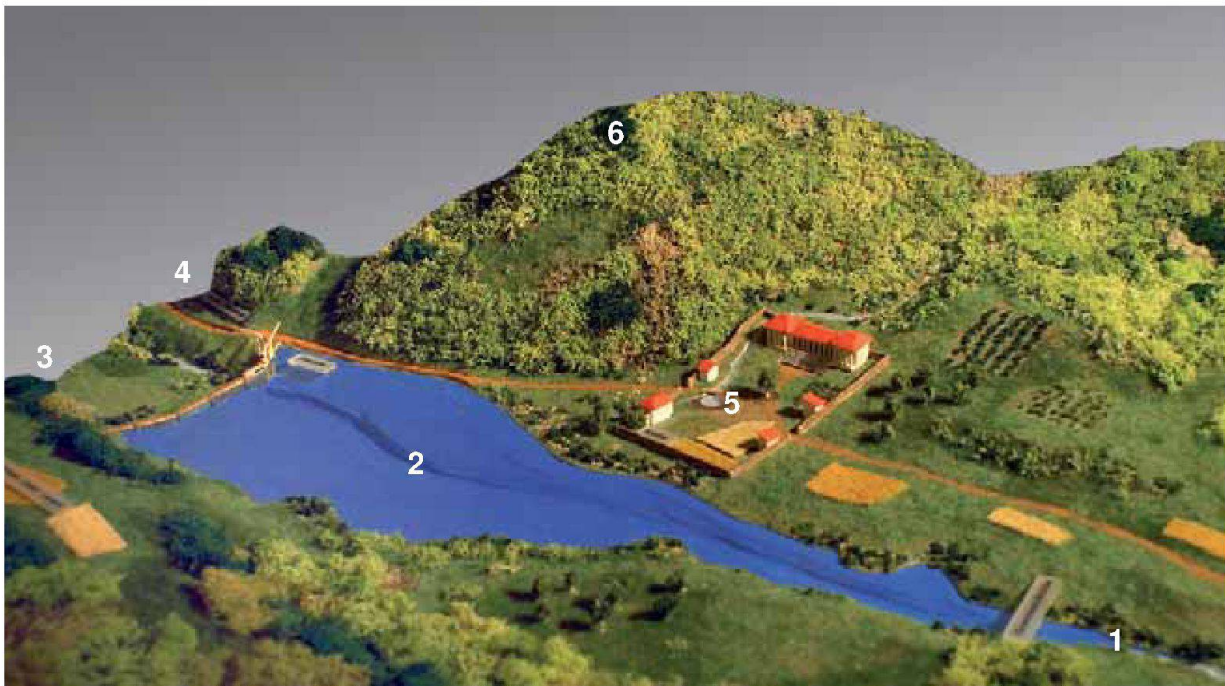
Abb. 35: Lausen-Bettenach, 6,6 km oberhalb von Augusta Raurica. Zufälligerweise baute Georg Schmid etwa zur selben Zeit ein Modell des postulierten Wasserefassungs-Stausees für eine Ausstellung im Ortsmuseum Lausen, wie die Planskizze von Markus Schaub (Abb. 34) entstand. Zu erkennen sind 1 die von Osten (rechts) kommende Ergolz, 2 der postulierte antike Stausee, 3 das tief gelegene Bett der Ergolz Richtung Westen (Liestal, Augst/Rhein), 4 die Wasserefassung und das Anfangsstück der römischen Wasserleitung (vgl. den untersten Abschnitt Abb. 48), 5 der archäologisch nachgewiesene römische Gutshof Lausen-Bettenach und 6 der Hügelzug «Plänezen» (zur Topografie siehe Abb. 34).
