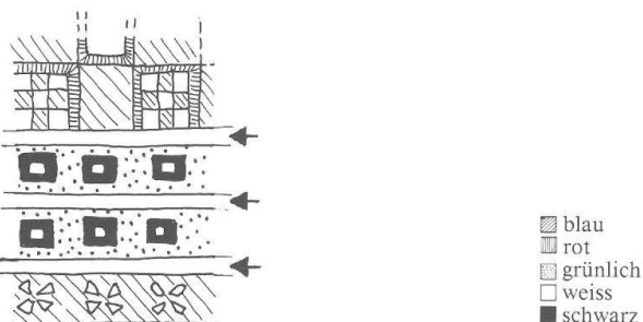
Abb. 5 Augst/Kaiseraugst, Kat.-Nr. 2. Einlegeschema des Millefiorimosaiks. Die Pfeile auf der Zeichnung zeigen die Bronzelege zwischen den Mosaikteinlagen an. M. 2:1.
