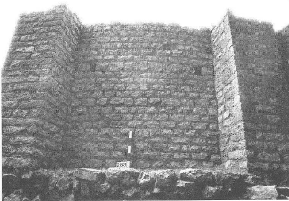
Abb. 17 Augst BL, Osttor. Grabung 1991.52. Blick gegen Süden an die Umfassungsmauer 7, zwischen den beiden Stützpfeilern 34 (rechts) und 35 (links). Wie bei der Ost- stützmauer 8 (Abb. 2) sind die Pfeiler auch beim Grabmonument mit Sandsteinbin- dern versehen (Abb. 18). Man beachte auch die zwei Gerüstlöcher in der Umfassung- mauer.
