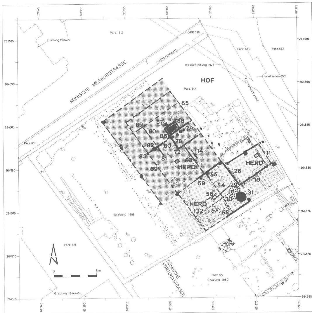
Abb. 25 August, Insula 22 (Grabung 1988.51), Bauzustand 3. M. 1:250.
