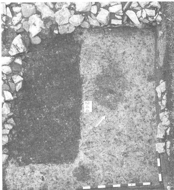
Abb. 57 Augst, Insula 22 (Grabung 1988.51), Zone 3, Bauzustand 1: Grube 94, «Arbeitsgrube» eines Schmiedes gefüllt mit Schmiedeaabfall (Hammerschlag). Verfüllte muldenförmige Vertiefung 96 am rechten Grubenrand. M. etwa 1:30.
