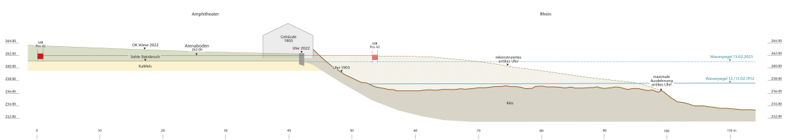
G: Kaiserstuhl AG, Bestandsaufnahme Amphitheater (Sondierung 2022.013). Umsetzung des Rheinprofil P 35 von 1912 mit Rheinwasserpegelständen und den Aufschüssen der Radomessur sowie der Reinschubbauwerke, M. 1:250.
