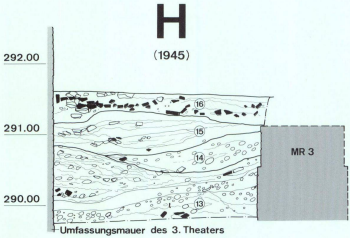
Beilage 2.H: Profil von 1945 (Grabung 1945.59). M. 1:40.
