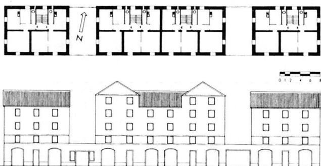
Fig. 59 Rue du Nord Nos 1–4, casernes locatives, 1871–1872. Plan de l'étage et élévation sur rue du Nord. Dessin G. Barbey. Extrait de Werk 63 (1976), p. 319.
