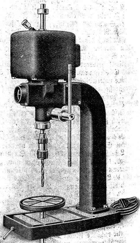
Abb. 1.2. Bohrmaschine mit direktem Motorantrieb (Werkstoff)
