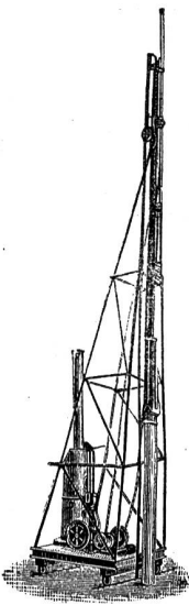
Rammarbeiten. [380 (M 10226 Z) Bestellgerichtete Gerüste auf Dielenunterlagen, Geleisen und Pontons.
