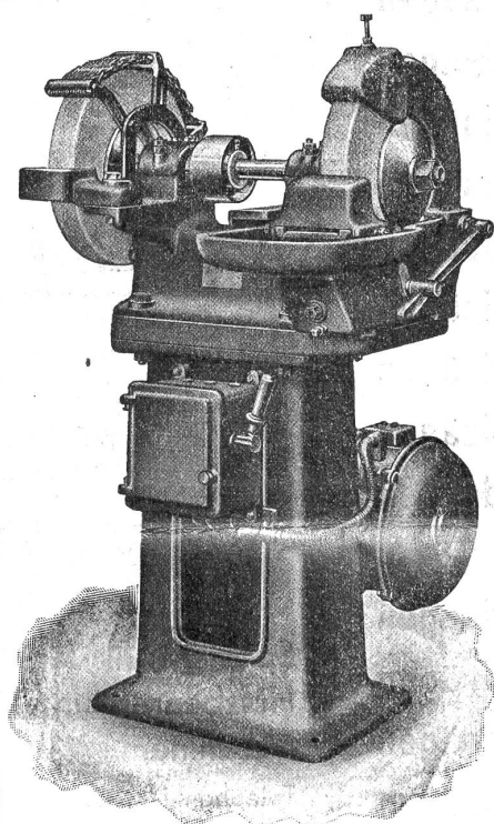
Mod. 30 b mit Einzelantrieb für Scheiben von 350×60 mm
