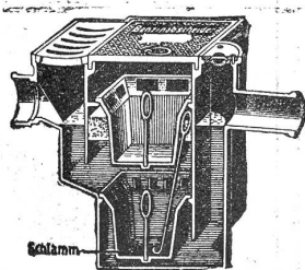
BENZIN-ABSCHIEDER
