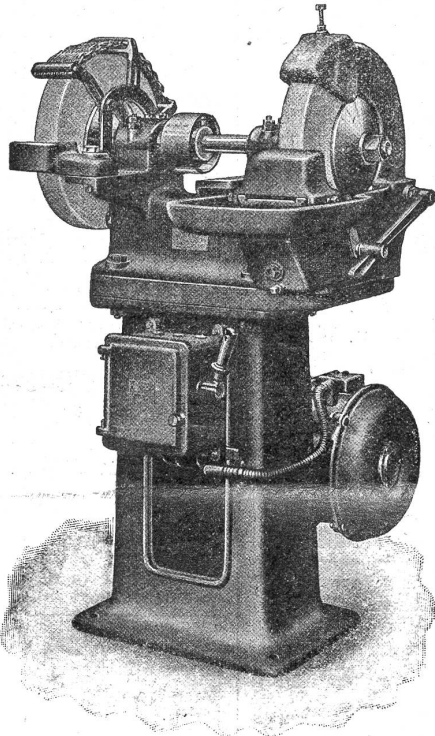
Mod. 30 b mit Einzelantrieb für Scheiben von 350×60 mm
