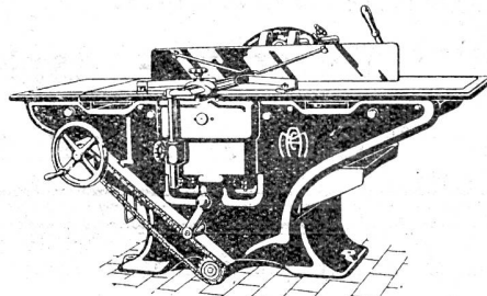
Kombinierte Abriht-, Kehl- und Dickenhobelmaschine 6 b Mod. H. D. — 360, 450, 530 und 610 mm Hobelbreite
