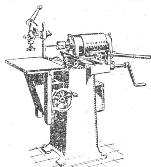
Riemenlose Langlochstochmaschine
