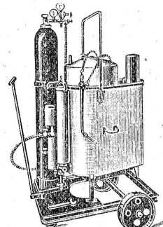
Grobstück-Apparat „Nova“
