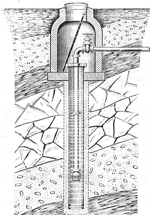
Rohrbruppen-Anlage System Reuther von 100–1850 mm l. W.
