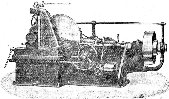
Schnell-Kaltsägemaschine SS.
