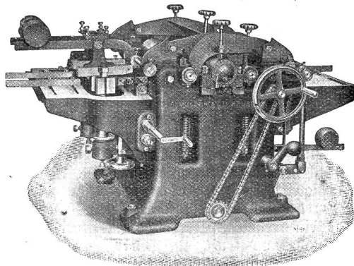
Dreiseitige Hobelmaschine.
