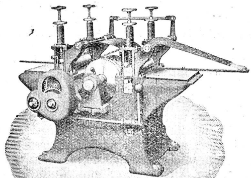
Latten-Kreissäge
