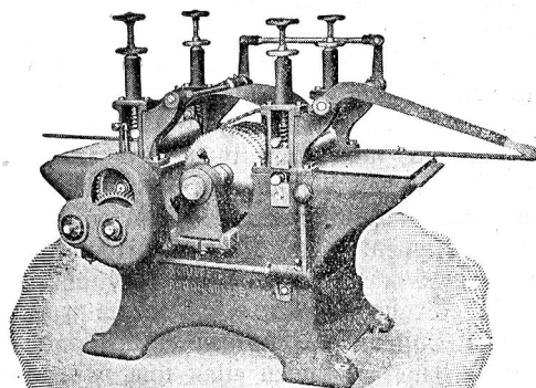
Latten-Kreissäge
