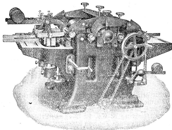
Dreiseitige Hobelmaschine.
