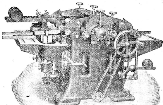
Latten-Kreissäge
