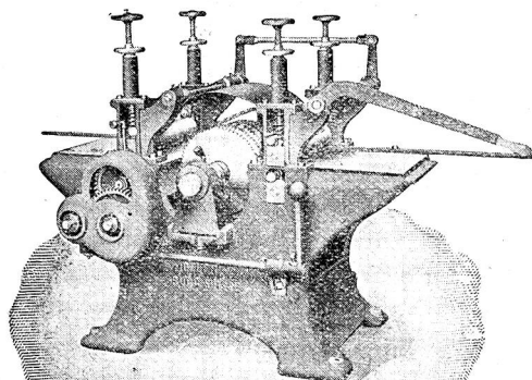
Latten-Kreissäge
