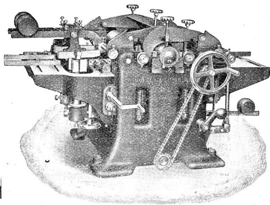
Dreseitige Hobelmaschine.
