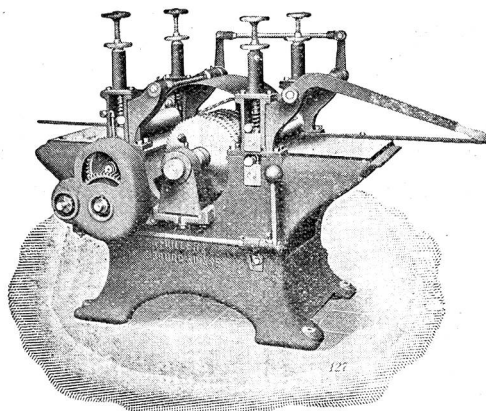
Latten-Kreissäge
