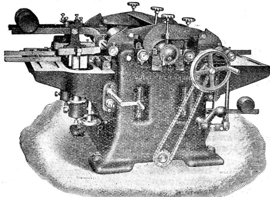
Dreiseitige Hobelmaschine.
