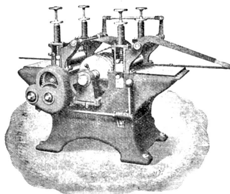
Latten-Kreissäge.
