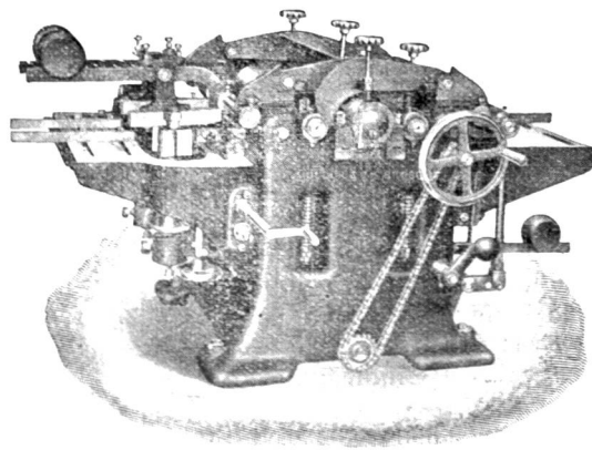
Dreiseitige Hobelmaschine.
