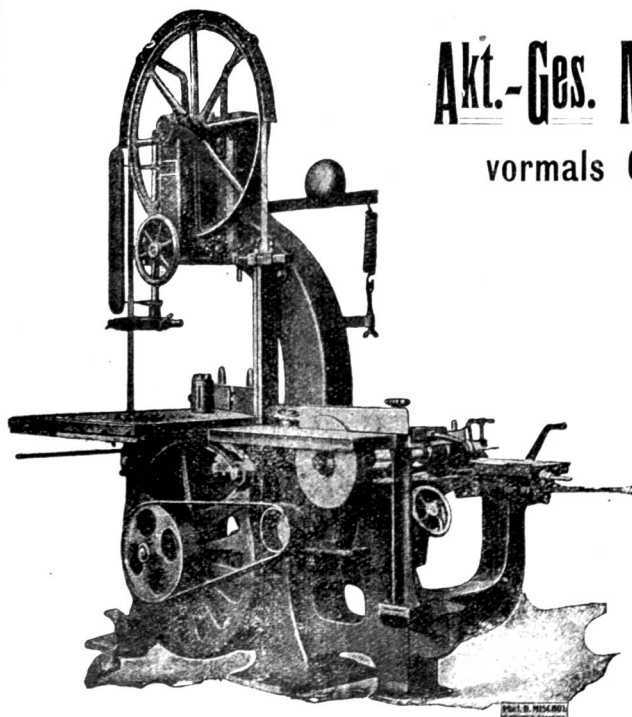
FUI. Neue Bandsäge mit Rollendurchmesser 800 mm kombiniert mit Kreissäge, Kehl- und Bohrmachine.
