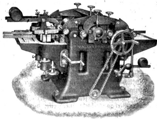
Dreiseitige Hobelmaschine.
