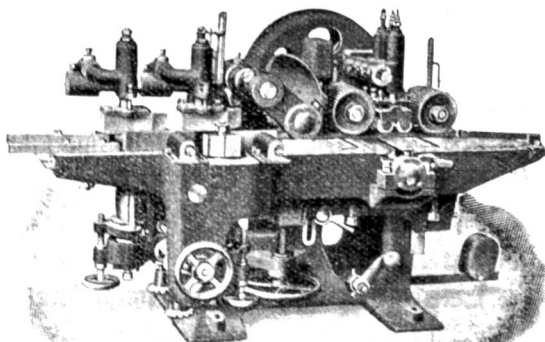
Vierseitige schmale Hobel- und Kehlmaschine.
