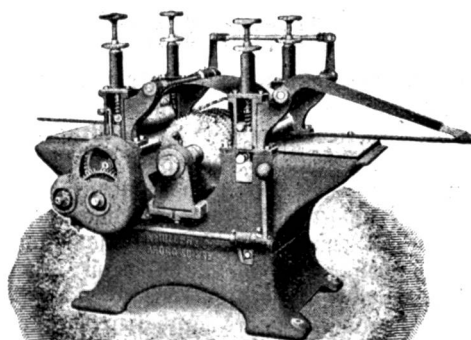
Latten-Kreissäge.
