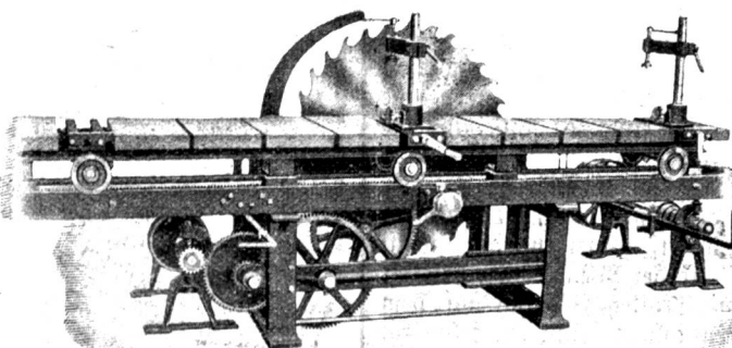
Kantholz- und Besäum-Kreissäge.
