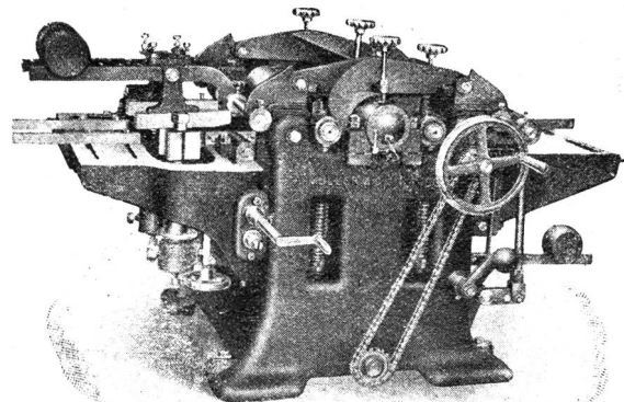
Dreiseitige Hobelmaschine.
