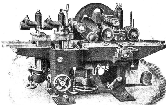
Vierseitige schmale Hobel- und Kehlmaschine.
