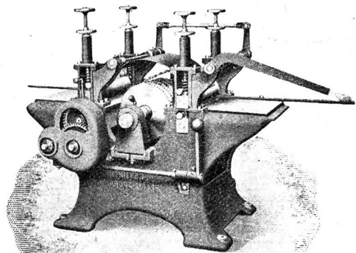
Latten-Kreissäge.
